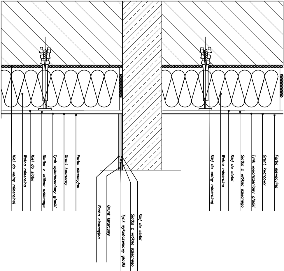
DETAL OCIEPLENIA ŚCIANY PRZY POŁĄCZENIU Z BALKONEM PRZEMÓJ POZIOMY
