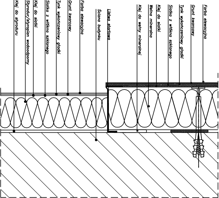
DETAL DOLNEJ KRAWĘDZI OCIEPLENIA PRZEMÓJ PIONOWY
