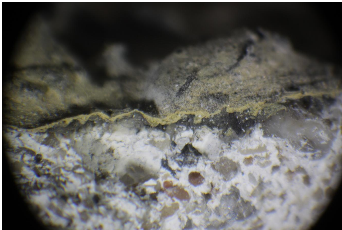
FOT. 21 - Mikroskopowy obraz fragmentu przekroju próbki nr 2
