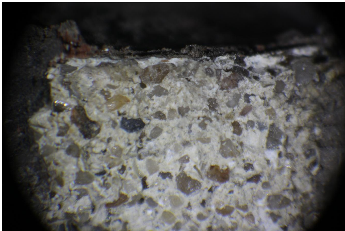
FOT. 20 - Mikroskopowy obraz fragmentu przekroju próbki pobranej ze spoiny muru, próbka nr 5
