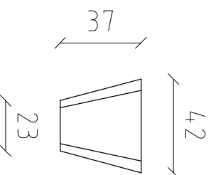
Z2 - Zwornik
