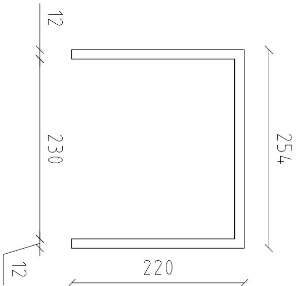
O1 - Opaska
